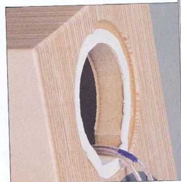
Durchdachte Verarbeitung: Die Holzschicht wird symmetrisch innen wie außen aufgesetzt – so werden alle Materialspannungen vermieden
